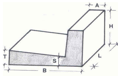
CORDOLO CUNETTA ALLA FRANCESE
