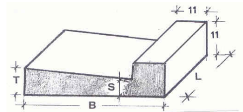
CORDOLO CUNETTA ALLA FRANCESE PER PASSO CARRABILE
