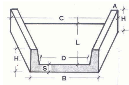
CUNETTA EMBRICE
